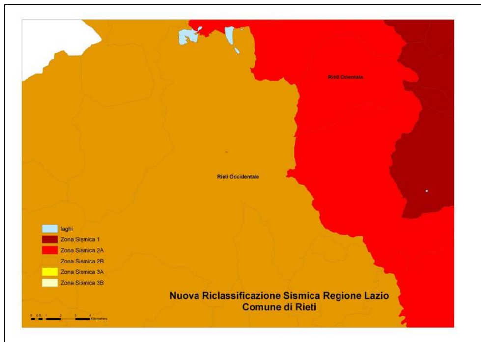
Riclassificazione Sismica del Comune di Rieti
